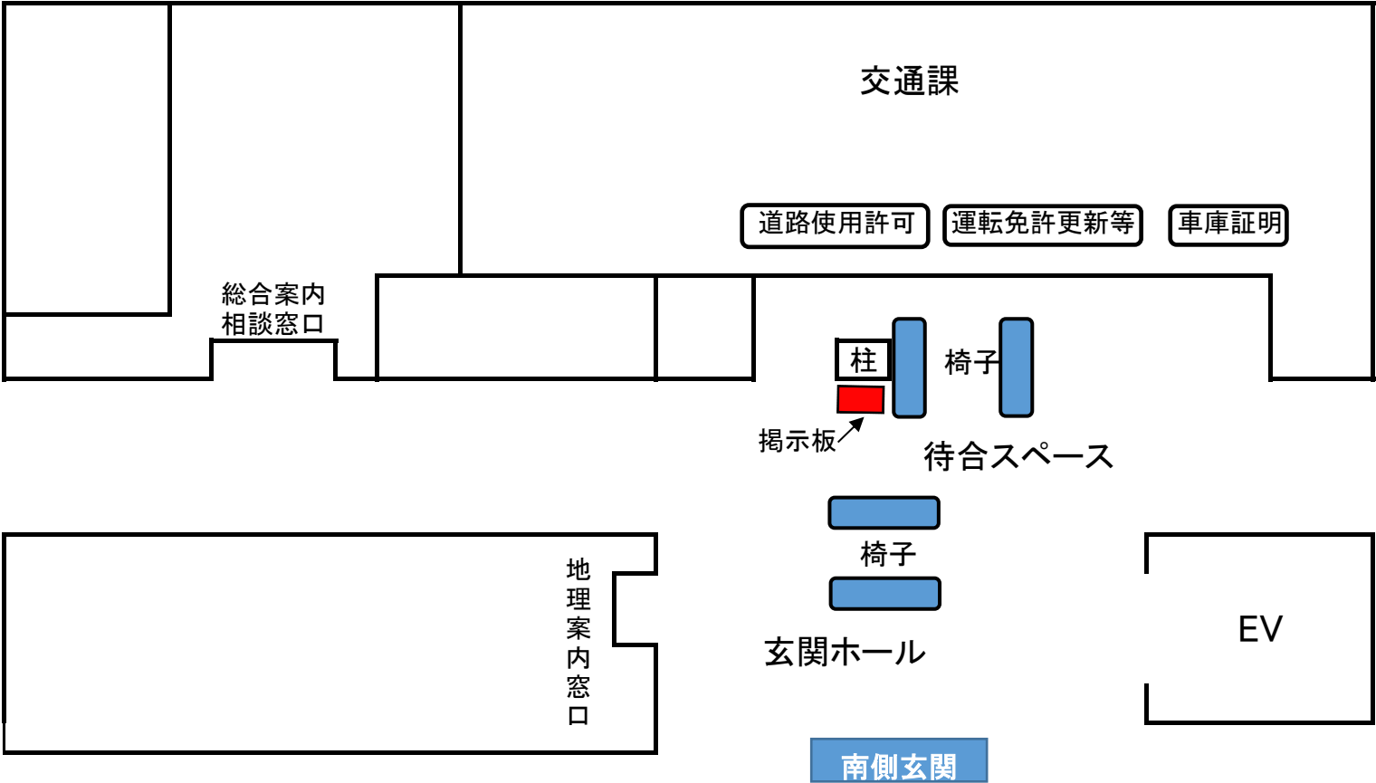
1階平面図
