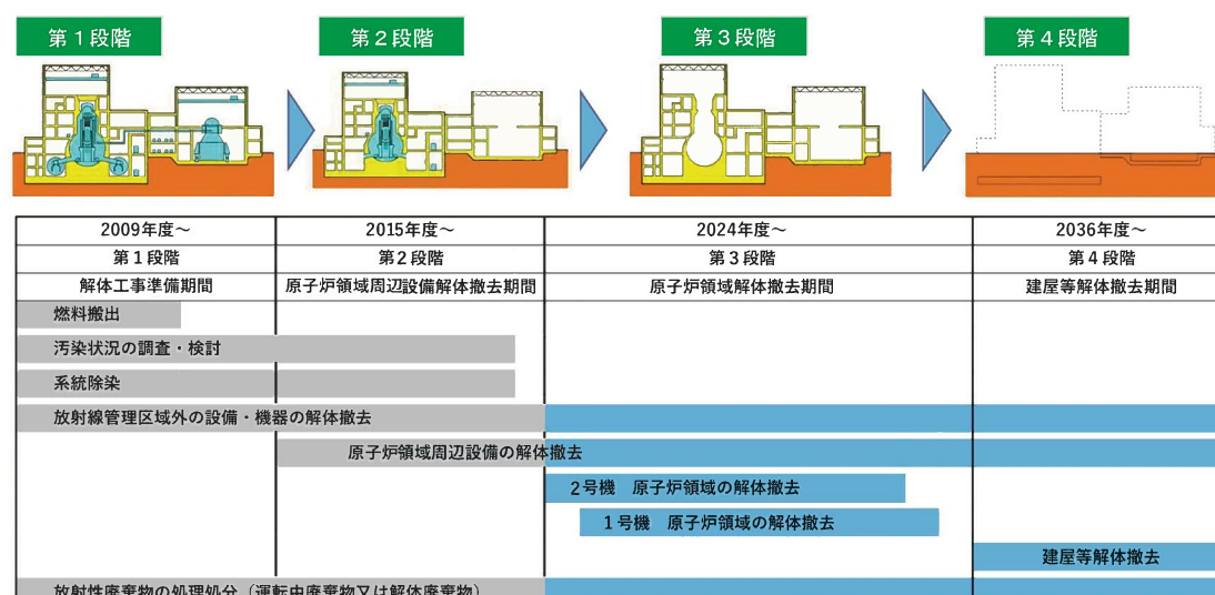
図 廃止措置の工程
