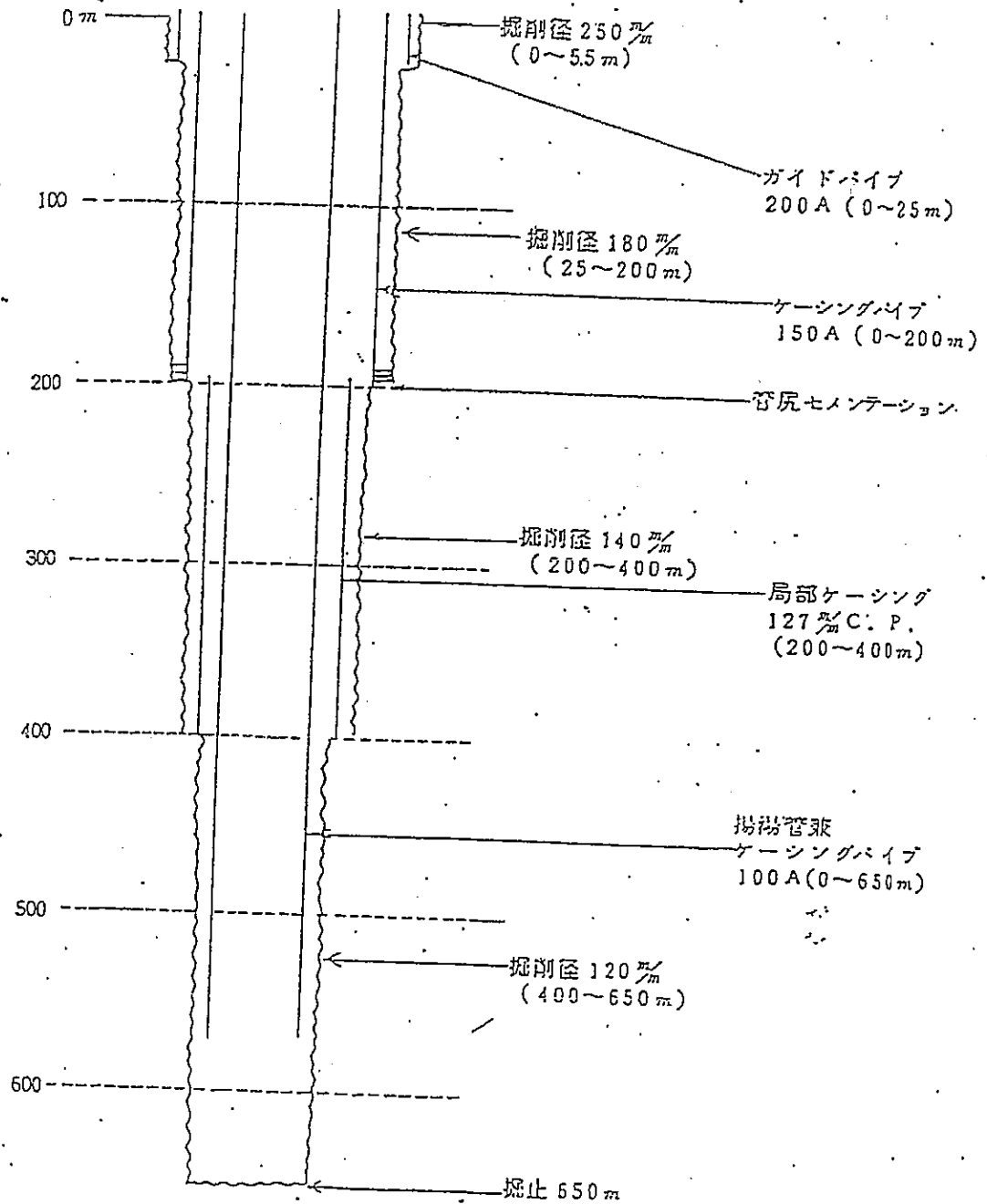
掘削孔仕上断面計画図 (例)
