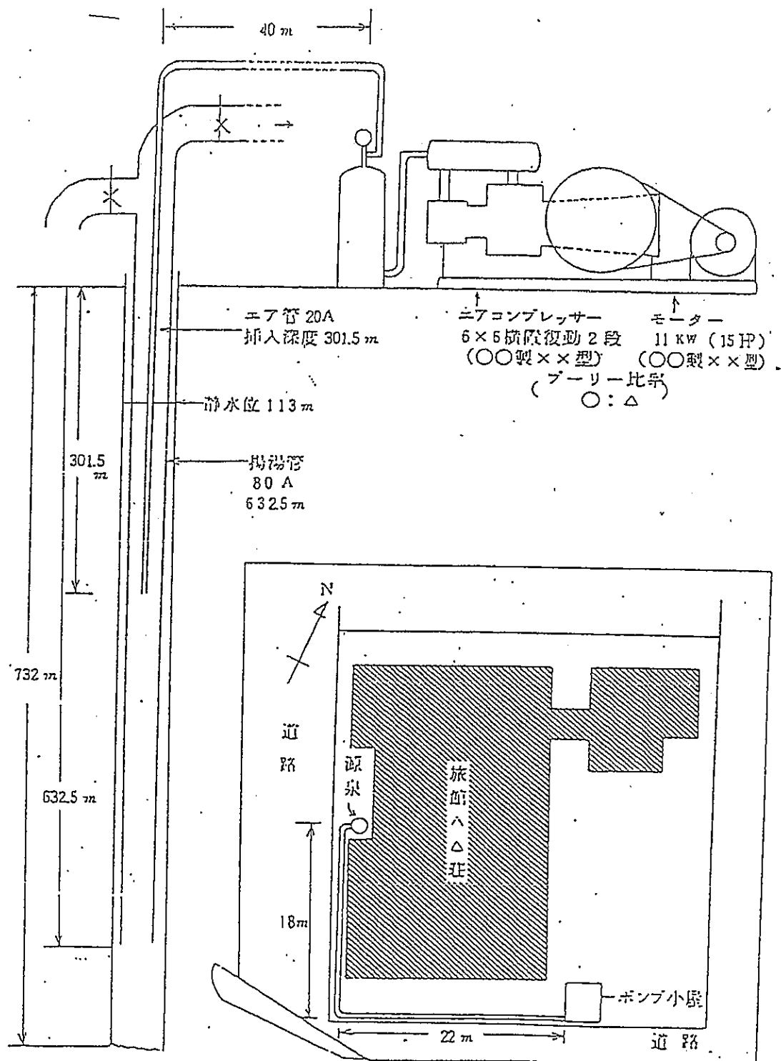
動力装置詳細説明図 (例)
