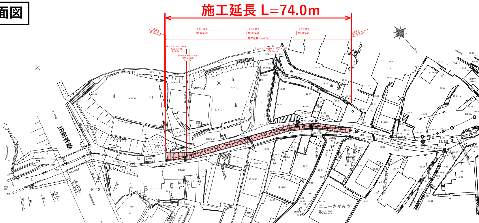
横断面図
