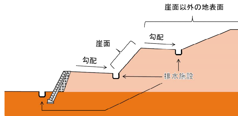
崖面と崖面以外の地表面のイメージ図
