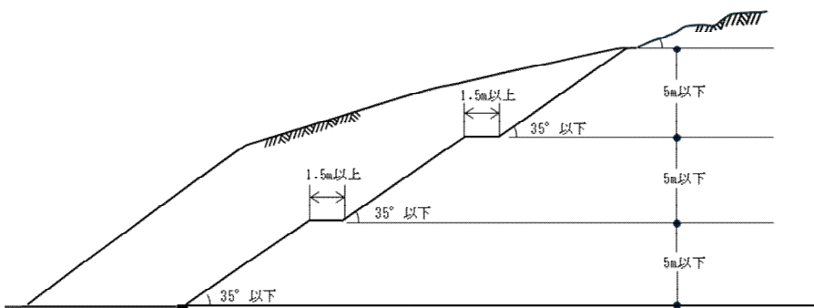
切土法面の形状（擁壁を設置しない場合） 砂利、真砂土、関東ローム、硬質粘土、富士マサ その他これらに類するもの
