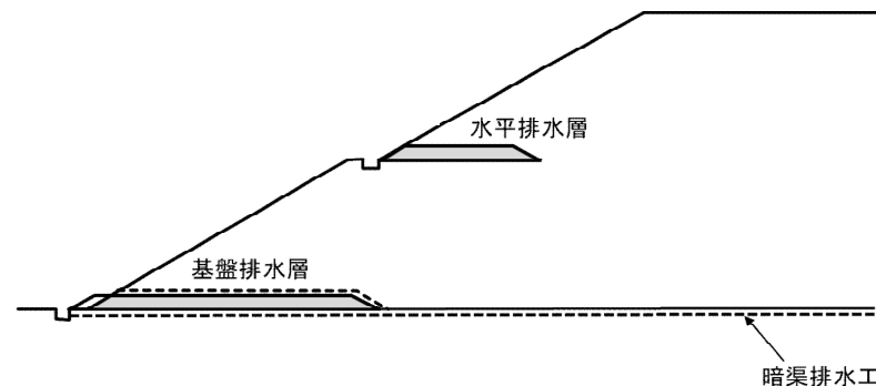
盛土の排水施設の概要図
