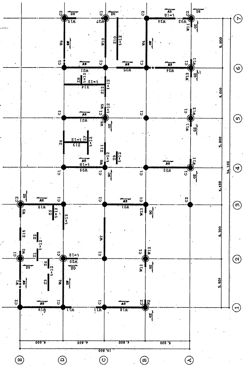
I 階伏図 SL. 1:200
