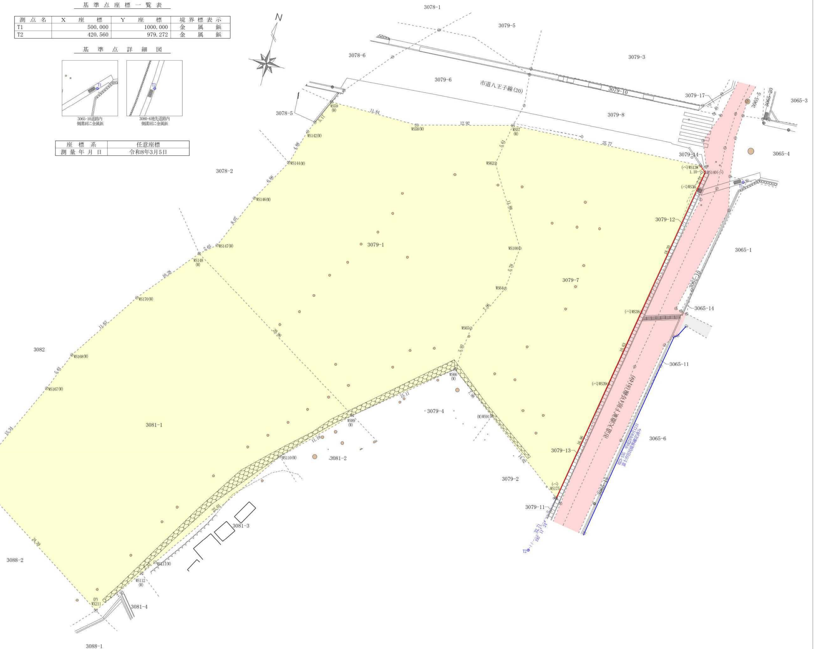
基準点座標一覧表
