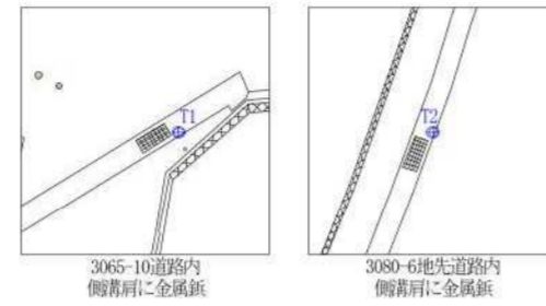
基準点詳細図
