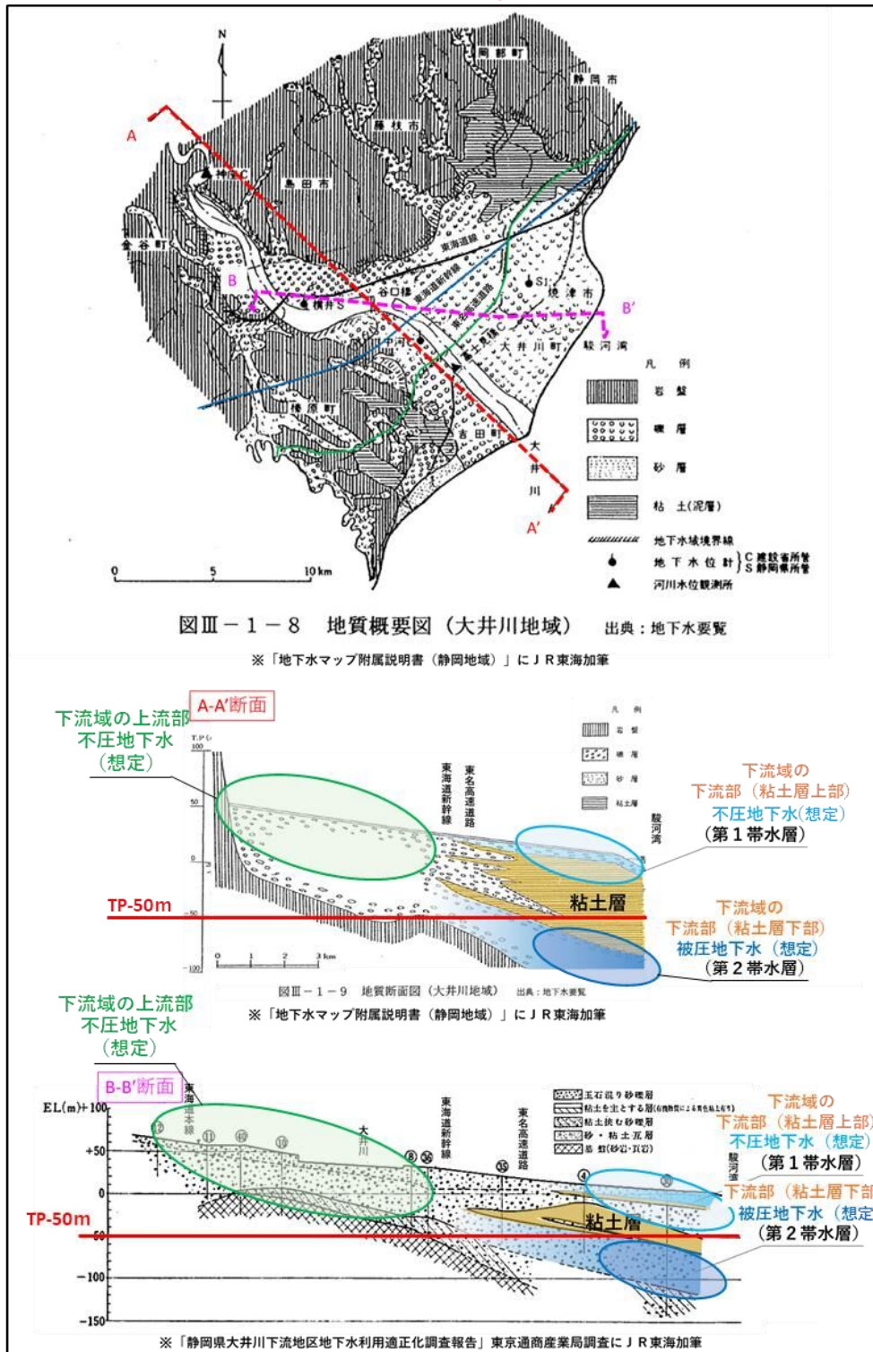
図 22 大井川下流域の帯水層調査結果（帯水層区分）
