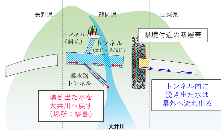
図1. 県境付近の断層帯を掘削中のトンネル湧水の流れ（イメージ）
