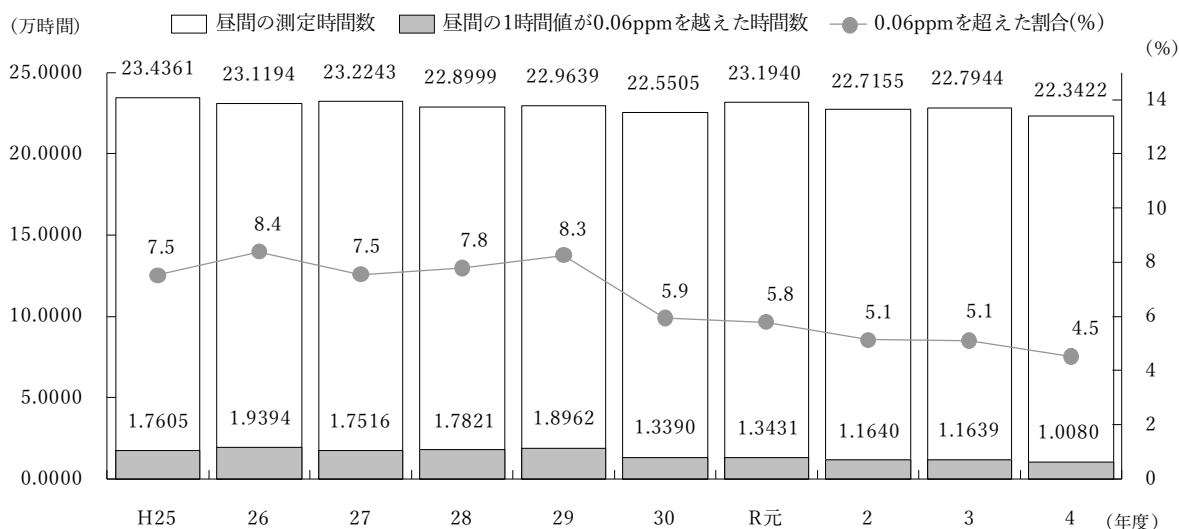
図Ⅱ－6 昼間の1時間値が0.06 ppm を超えた時間数の経年変化
