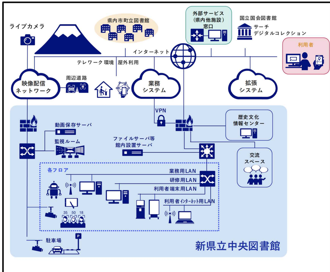
<参考：ネットワークイメージ> (基本構想 P33 : 図6.1.2)
