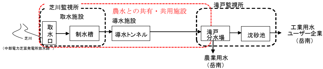
図表 2 旧富士川工業用水道の施設フロー
