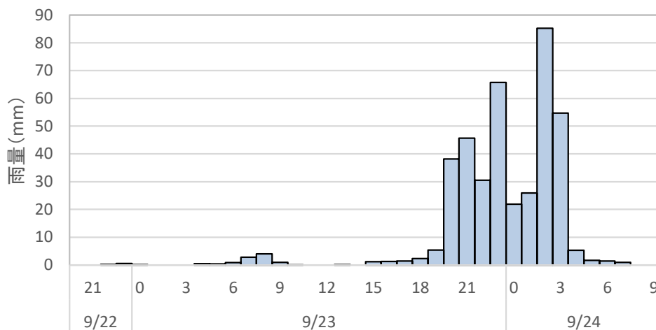
図 5.3 令和 4 年台風第 15 号に伴う豪雨
