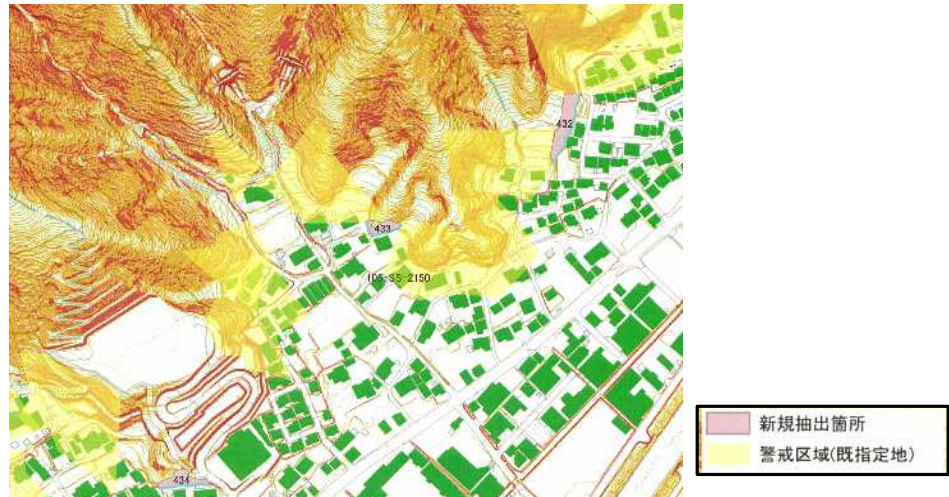
図 5.12 土砂災害警戒区域の抽出イメージ
