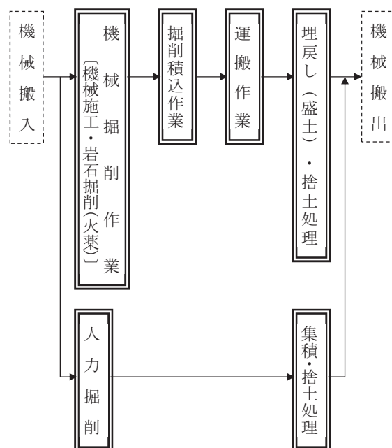
図2-1 施工フロー
