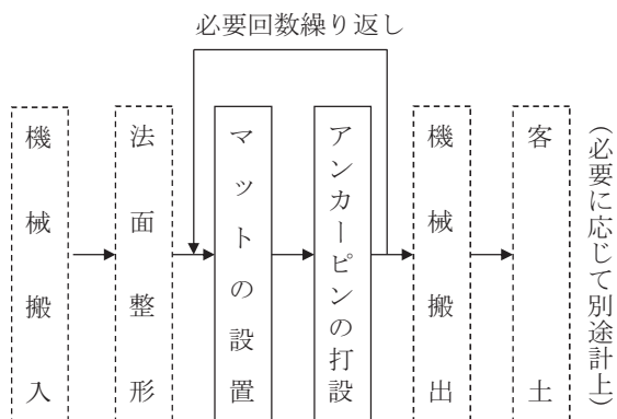
図2-1 施工フロー
