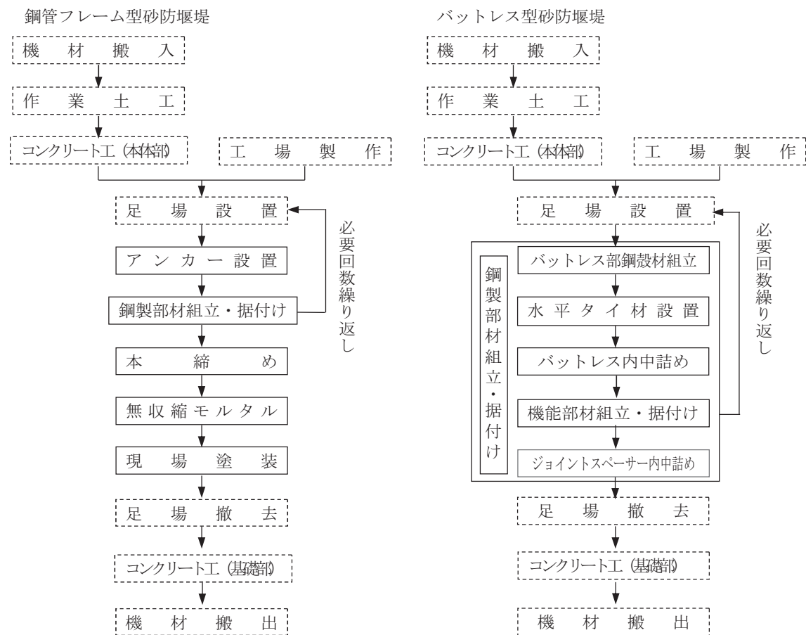
図2-1 施工フロー
