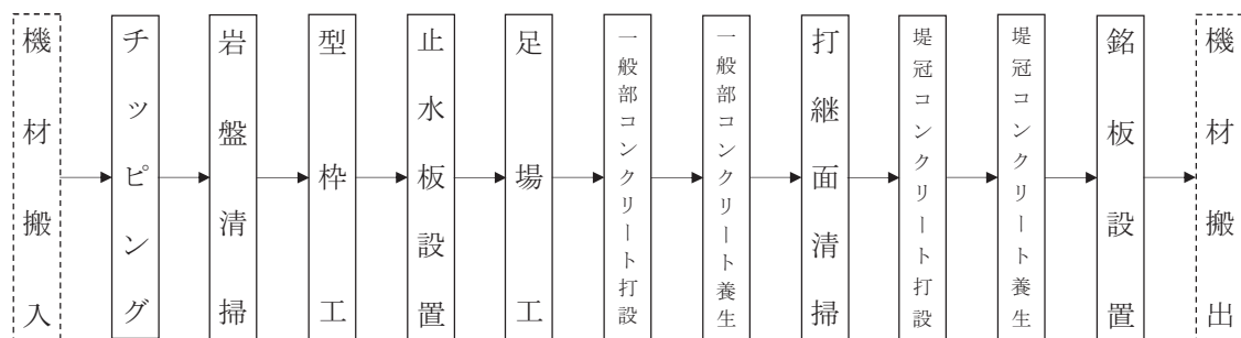
図2-1 施工フロー
