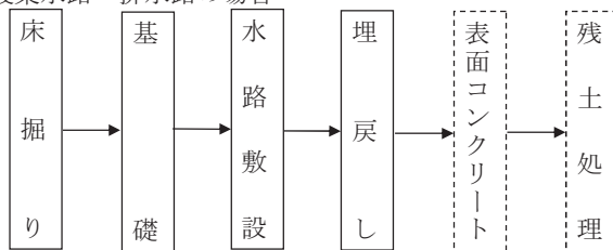
図2-1 施工フロー
