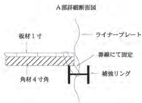
詳 細 図
