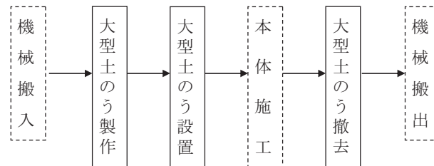
図 2-2 施工フロー
