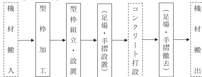
図2-1 施工フロー
