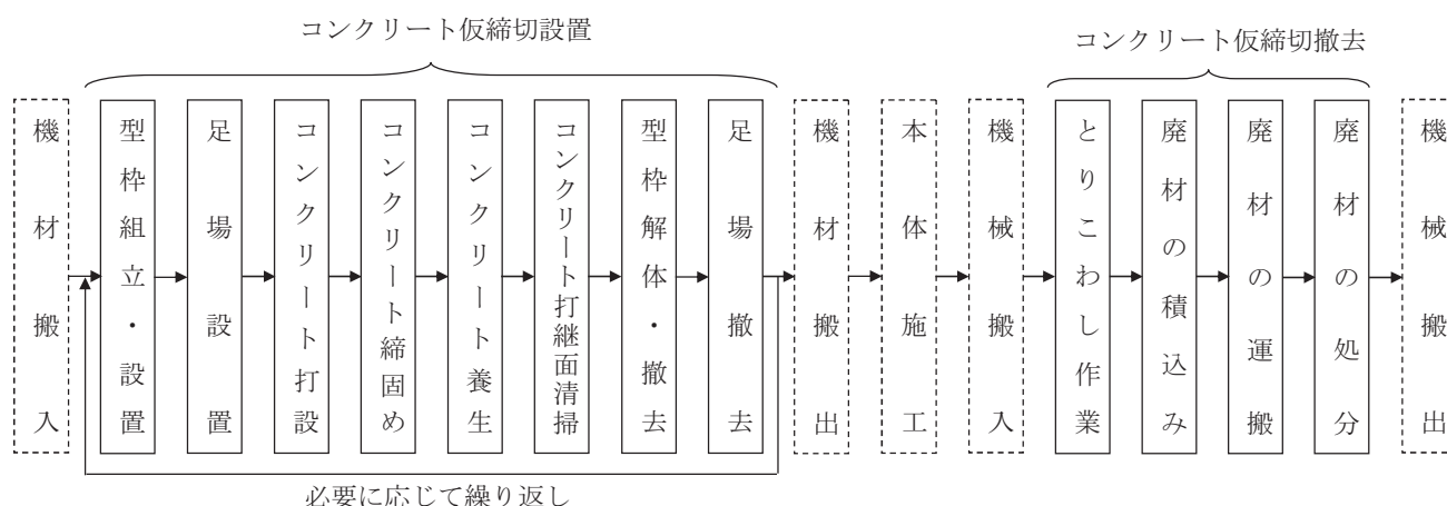
図2-1 施工フロー
