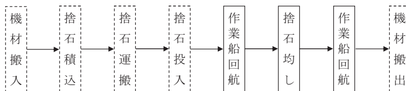
図2-1 施工フロー
