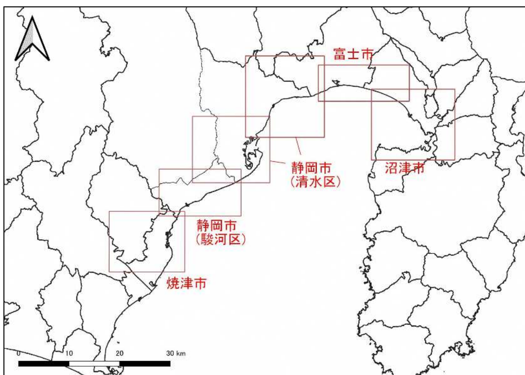
図 5-2 計算領域及び計算格子間隔 (2) (主な地域：焼津市、静岡市、富士市、沼津市 ※2 )
