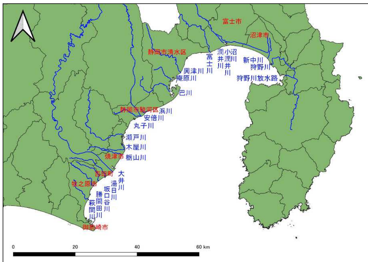
図 3-7 河川流量を考慮した河川
