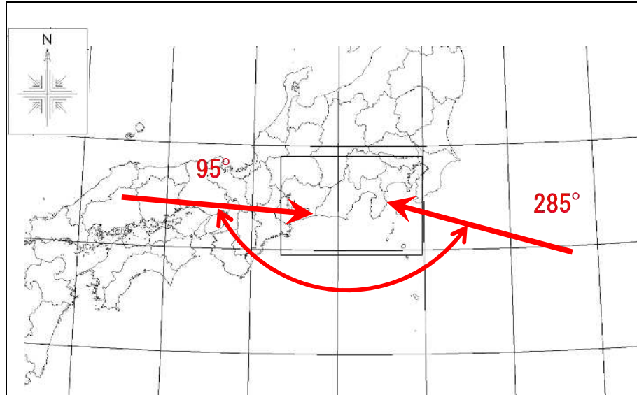
図 3-3 静岡県沿岸に影響する台風経路範囲
