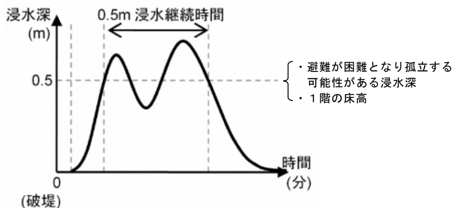
図 2-2 浸水継続時間
