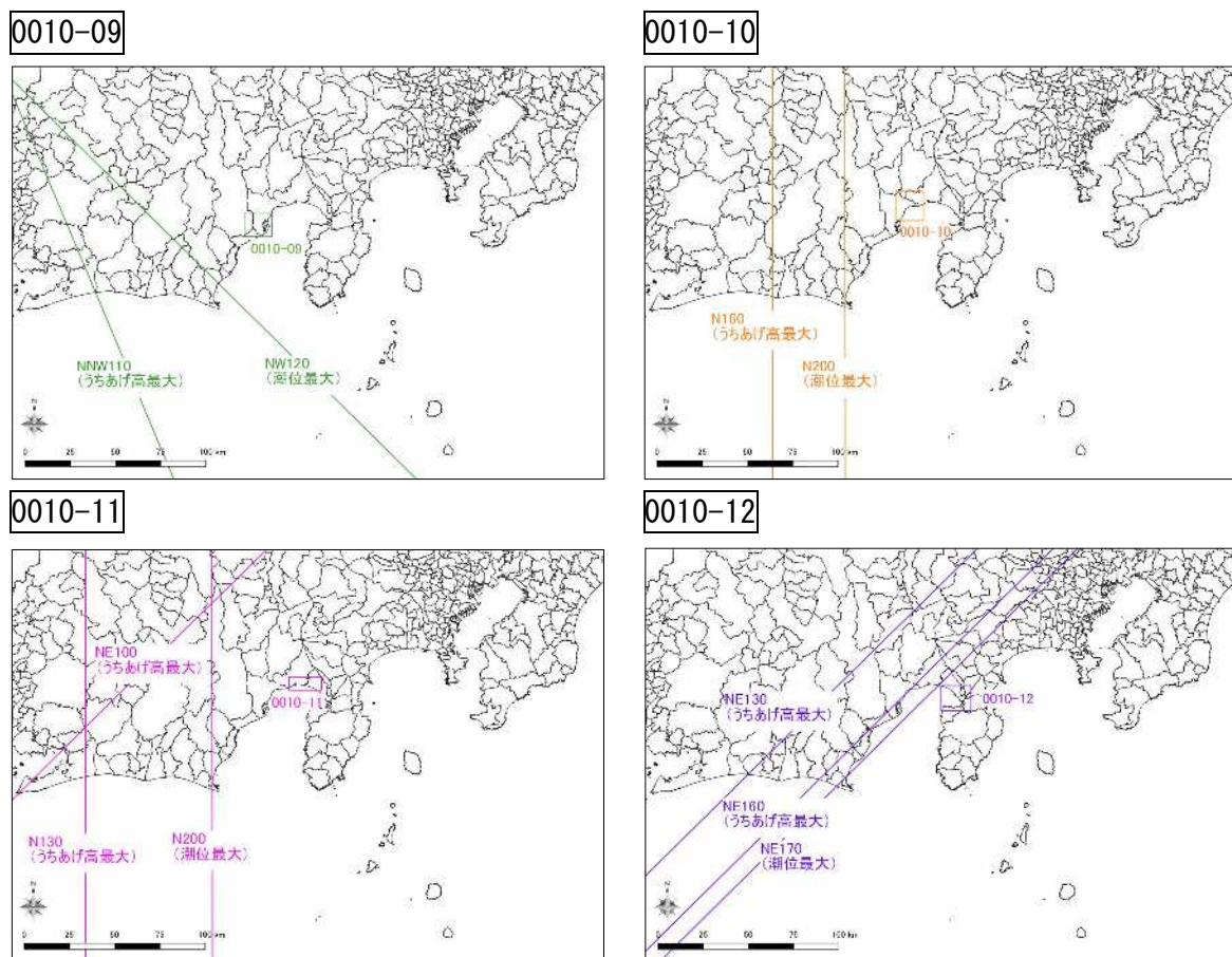
図 3-4 各計算領域における危険となる台風経路
