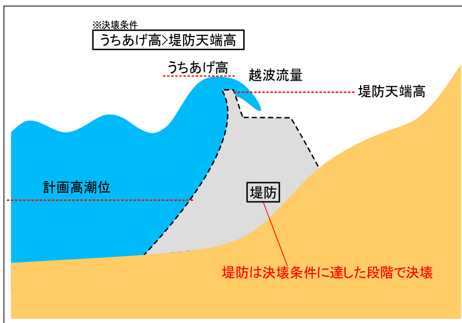
図 4-1 海岸堤防等の決壊条件のイメージ
