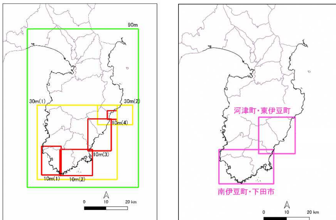
図 5-2 計算領域及び計算格子間隔 (2) (主な地域：南伊豆町、下田市、河津町、東伊豆町)
