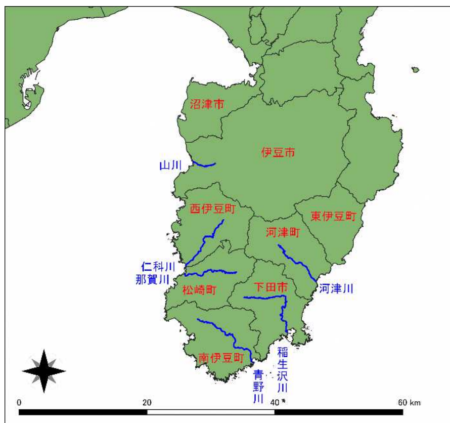
図 3-7 河川流量を考慮した河川
