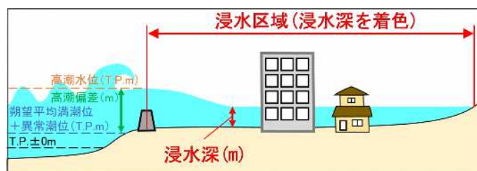
図 9-1 浸水区域と浸水深の定義
