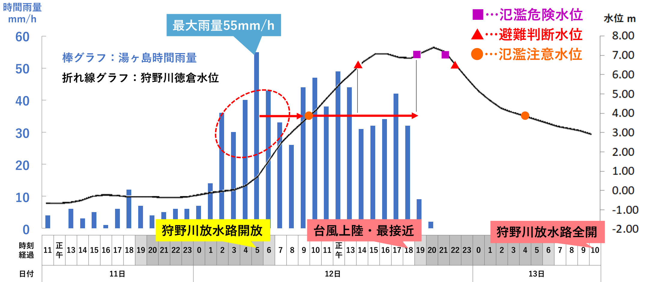
令和元年10月 台風19号 雨量・水位グラフと気象警報（狩野川流域市町）
