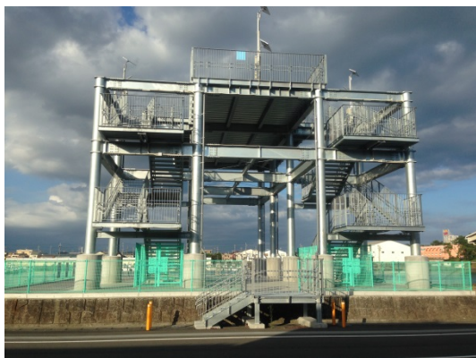
避難タワーの例（用宗漁港）
