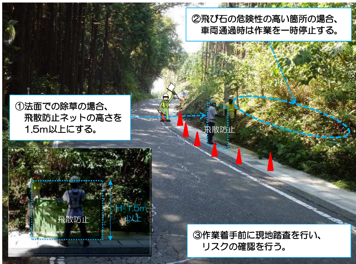
安全対策後の現場状況（イメージ）
