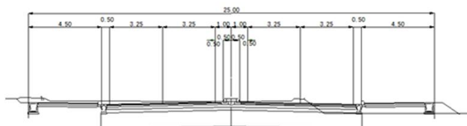
標準横断面図
