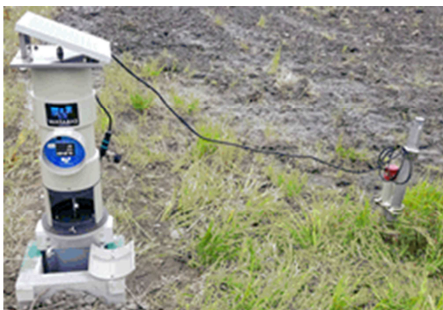
（自動給水栓（左）と水位計（右））
