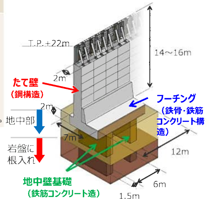
防波壁（一般部）の構造概要
