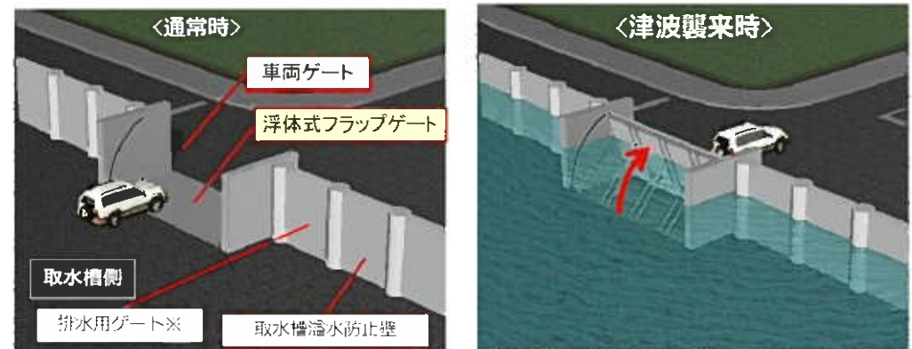
車両ゲートの構造概要（津波襲来時に自動閉鎖）
