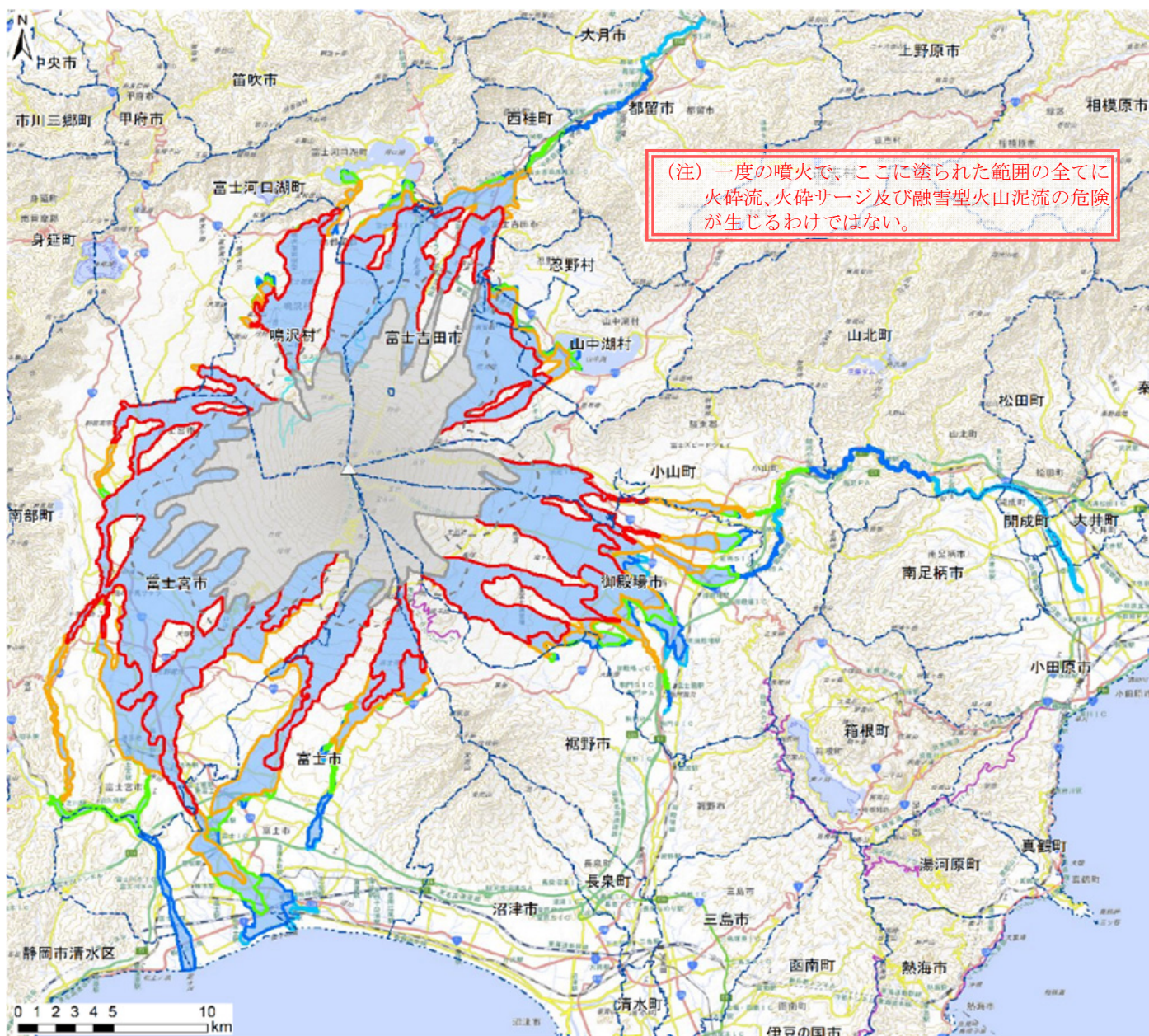
○ 融雪型火山泥流の可能性マップ（到達時間）（報告書_図 5.5-6）
