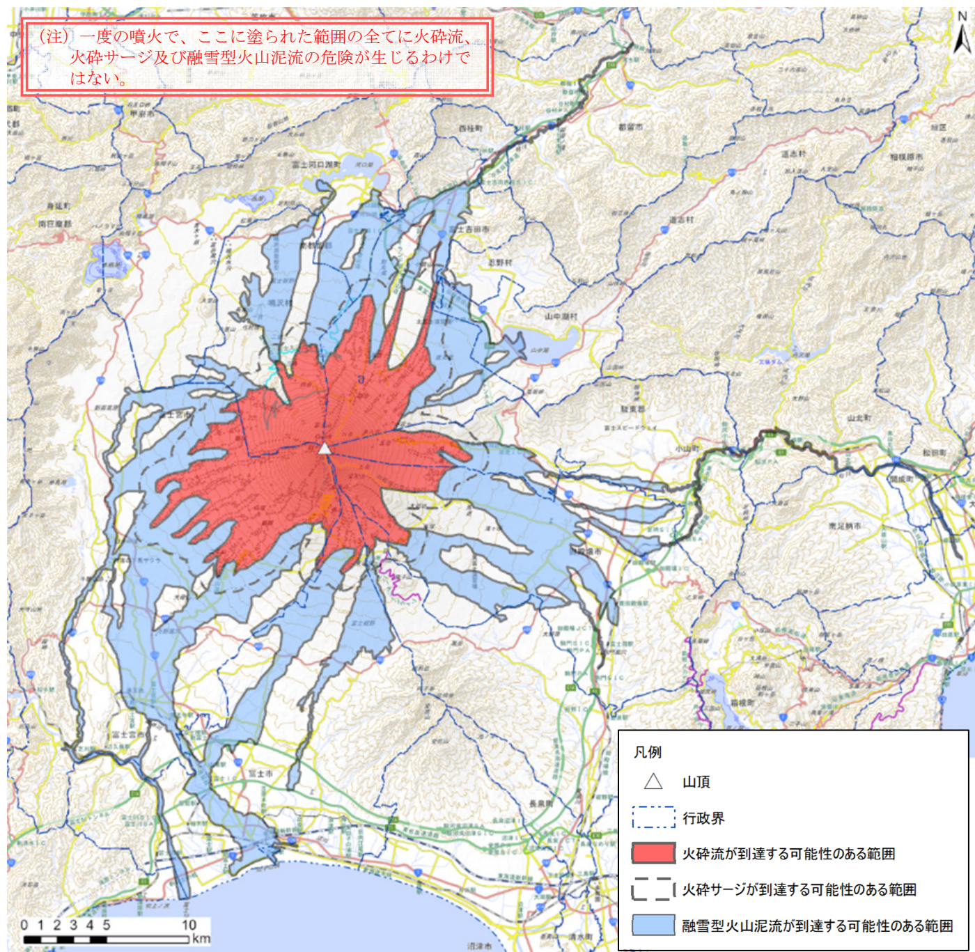
○ 融雪型火山泥流の可能性マップ（到達範囲）（報告書_図 5.5-5）
