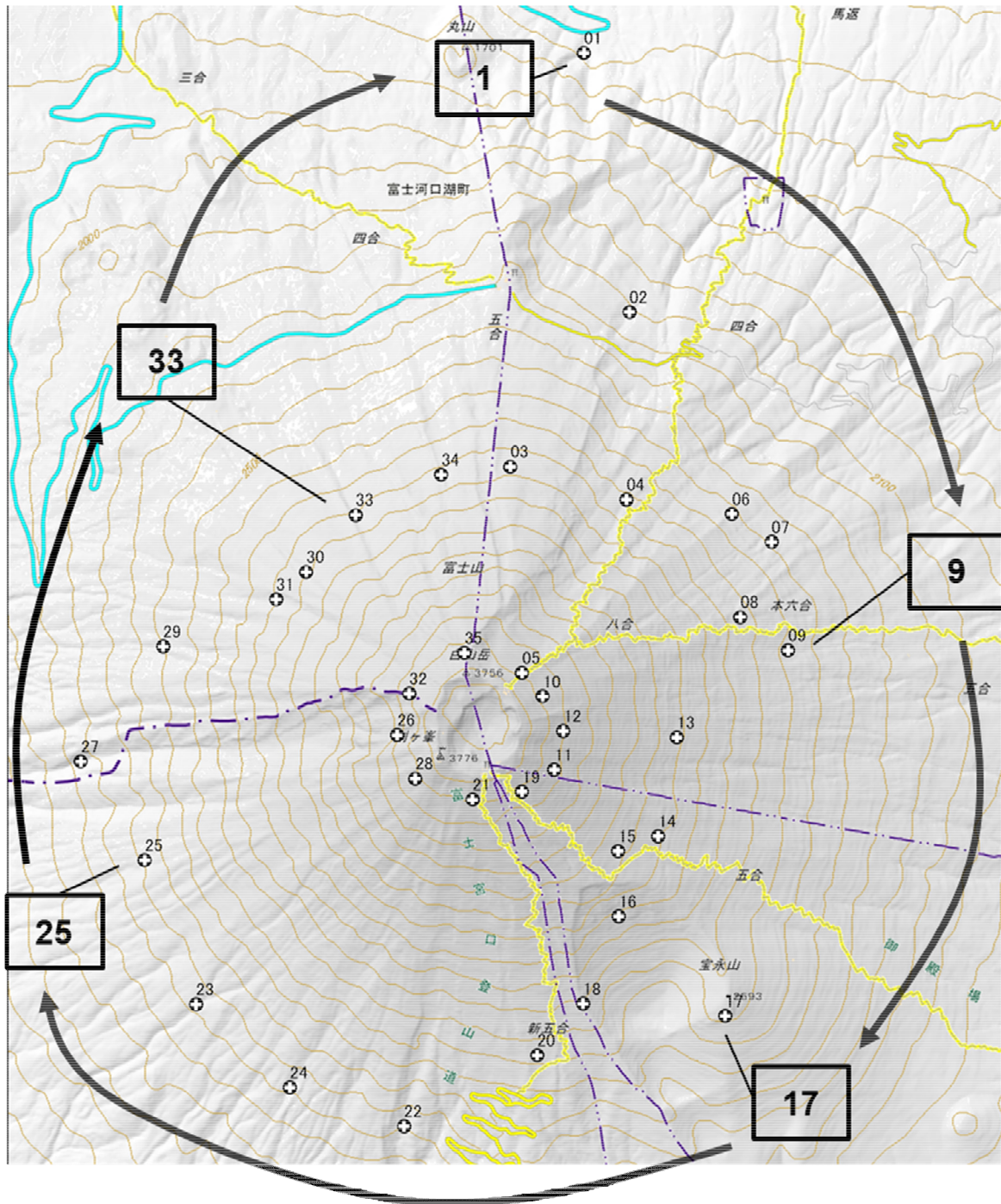
○ 火砕流のドリルマップ 計算開始点の配置一覧図（報告書_図 5.4-1）
