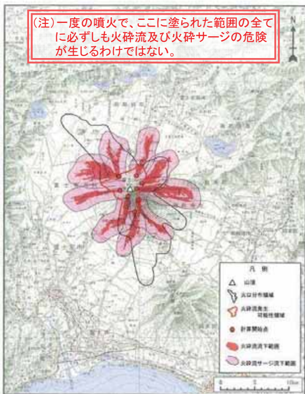
（旧） 火砕流のドリルマップ（平成16年版）
