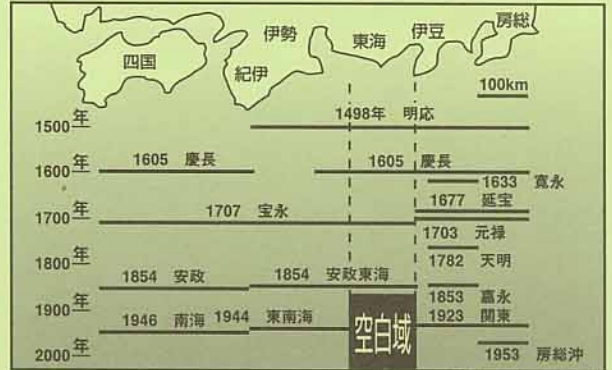
大太平洋岸で起こった過去の大地震
