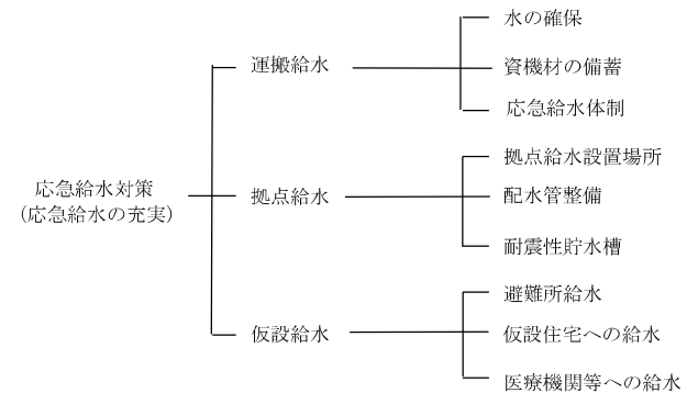
図 2.4.2.1 応急給水対策の分類
