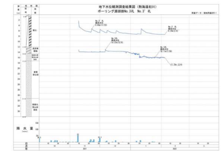
図 参-12 調査結果まとめ (ボーリング No. 3)
