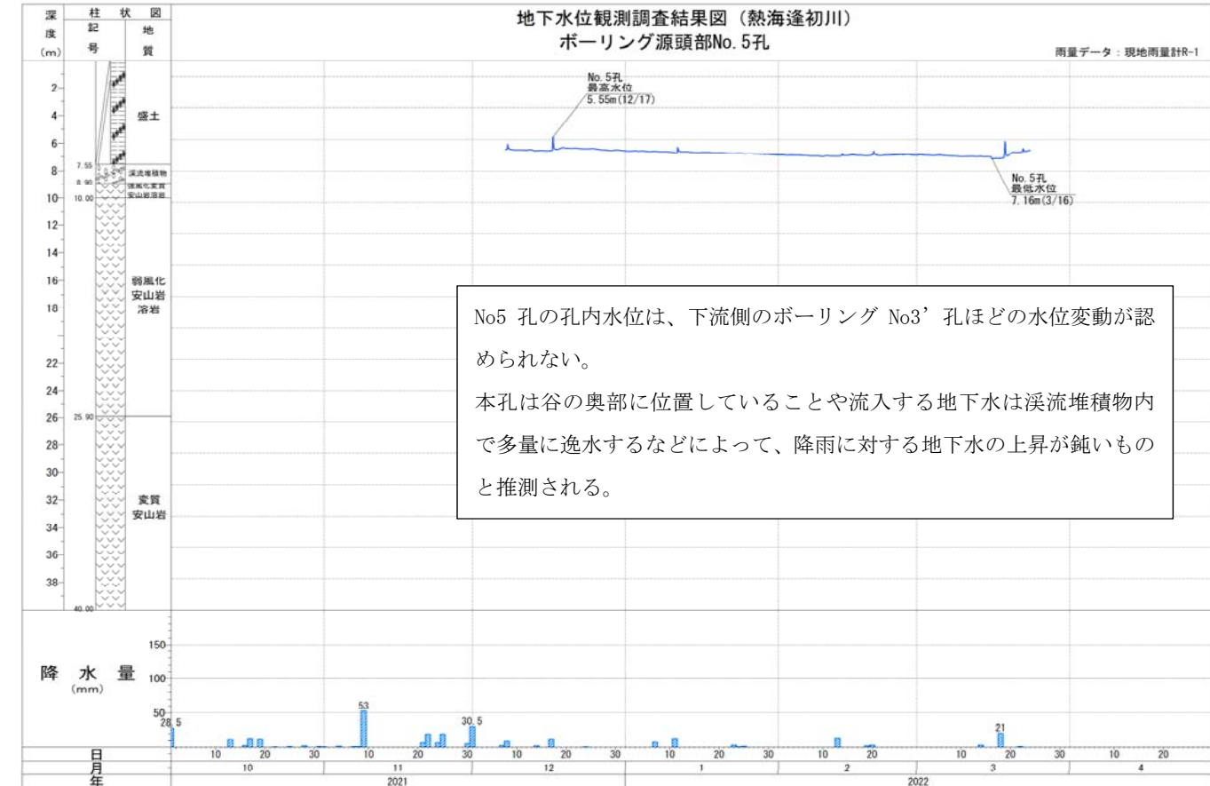
図 参-15 地下水位計結果（ボーリング No. 1, 2, 3, 5）
