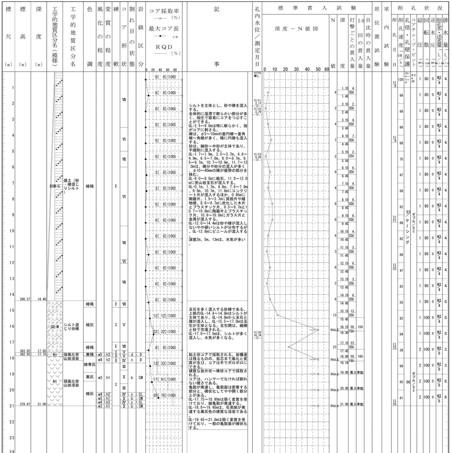
図 参-7 ボーリング柱状図 (No. 4)
