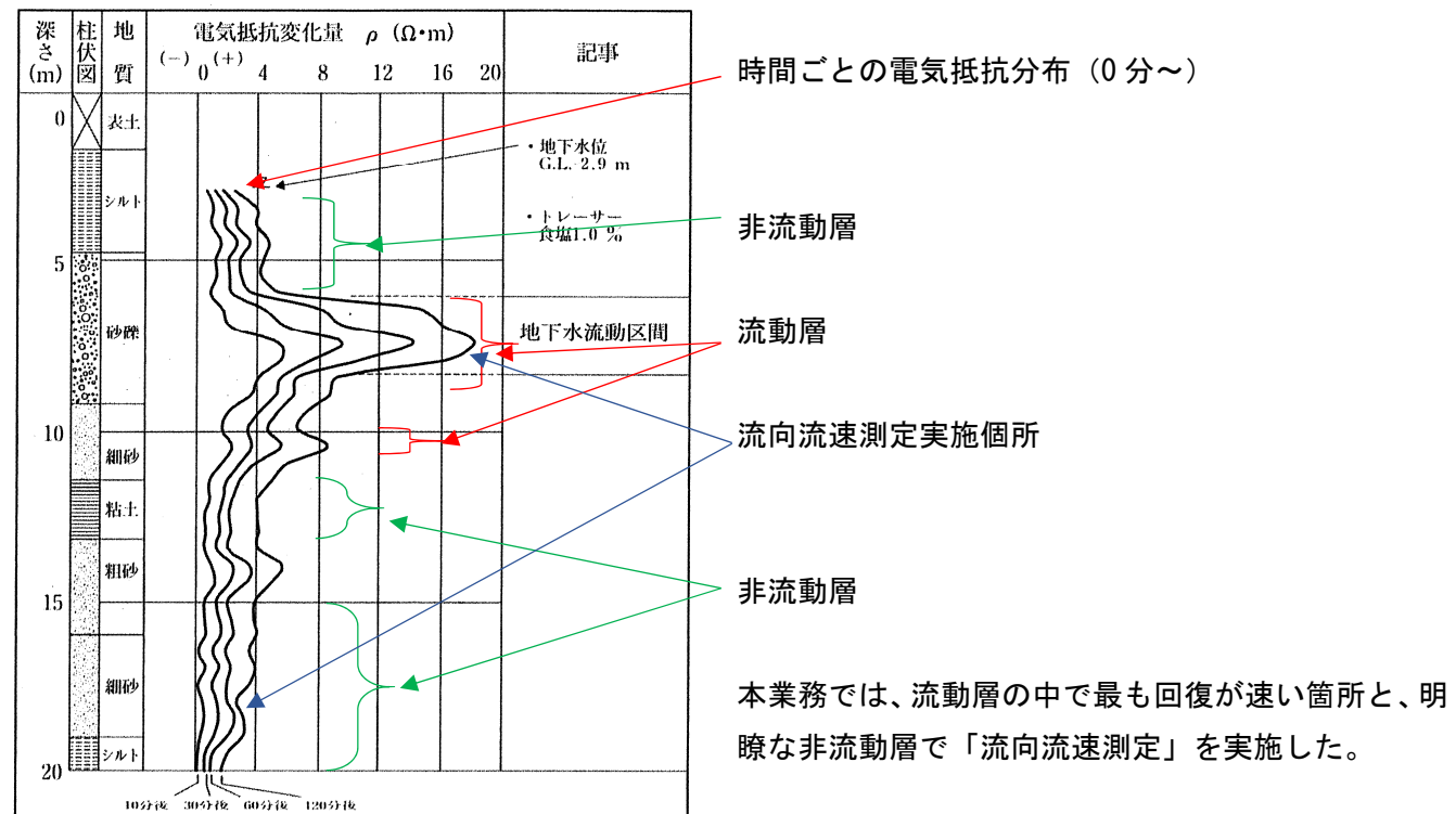
図参-16 地下水検層結果例
