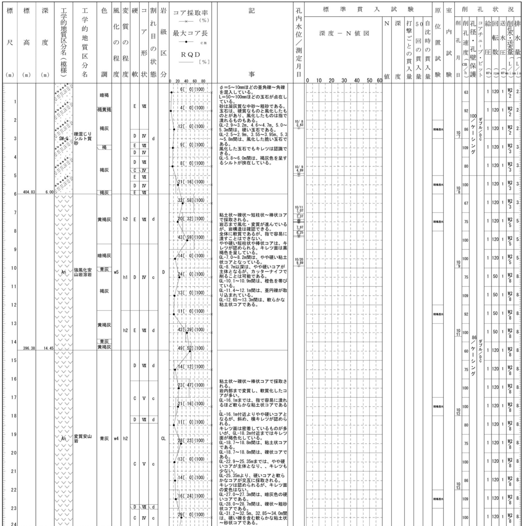
図 参- 3 ボーリング柱状図 (No. 2) (1/2)
