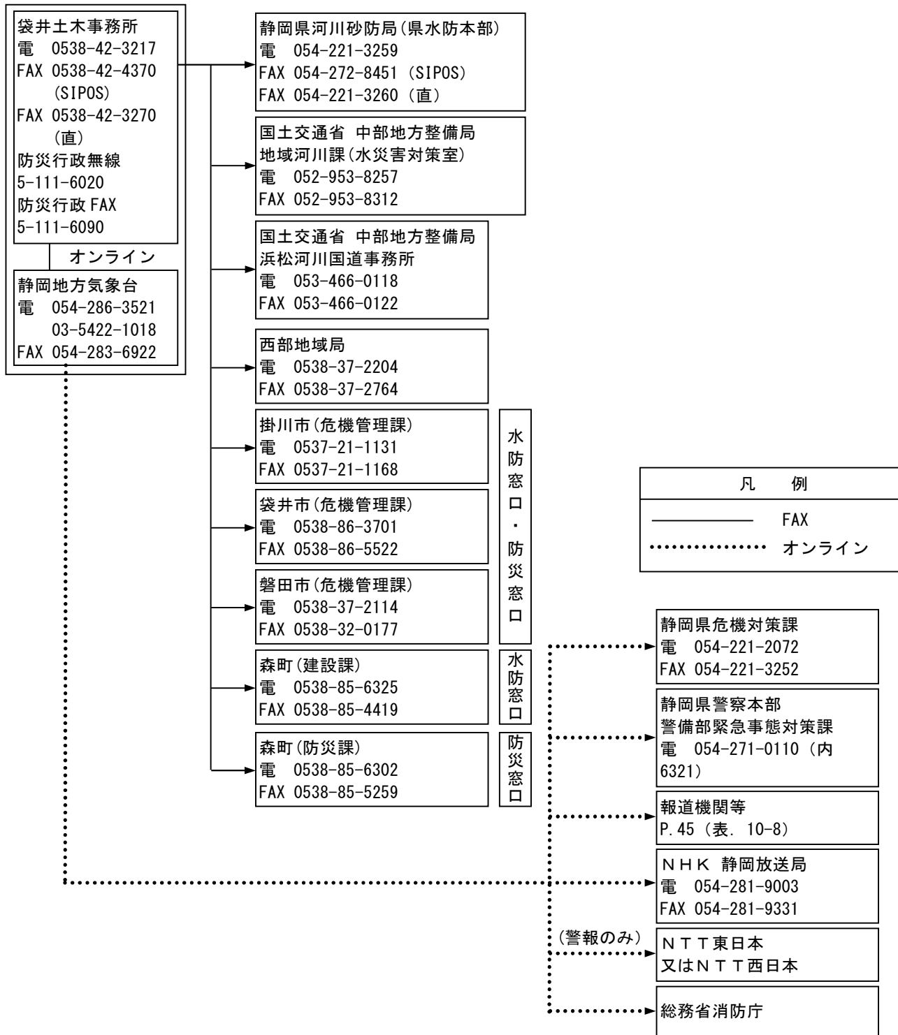
図. 10-8 太田川水系太田川・原野谷川洪水予報連絡系統図
