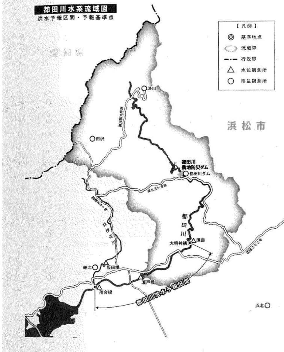
付図1 雨量・水位観測所配置図
