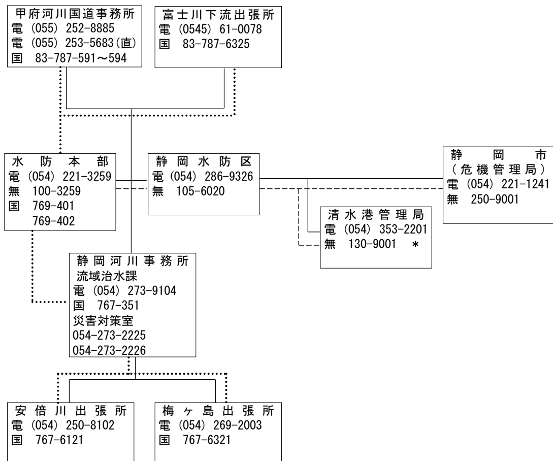
図. 16-5 静岡水防区連絡系統図
