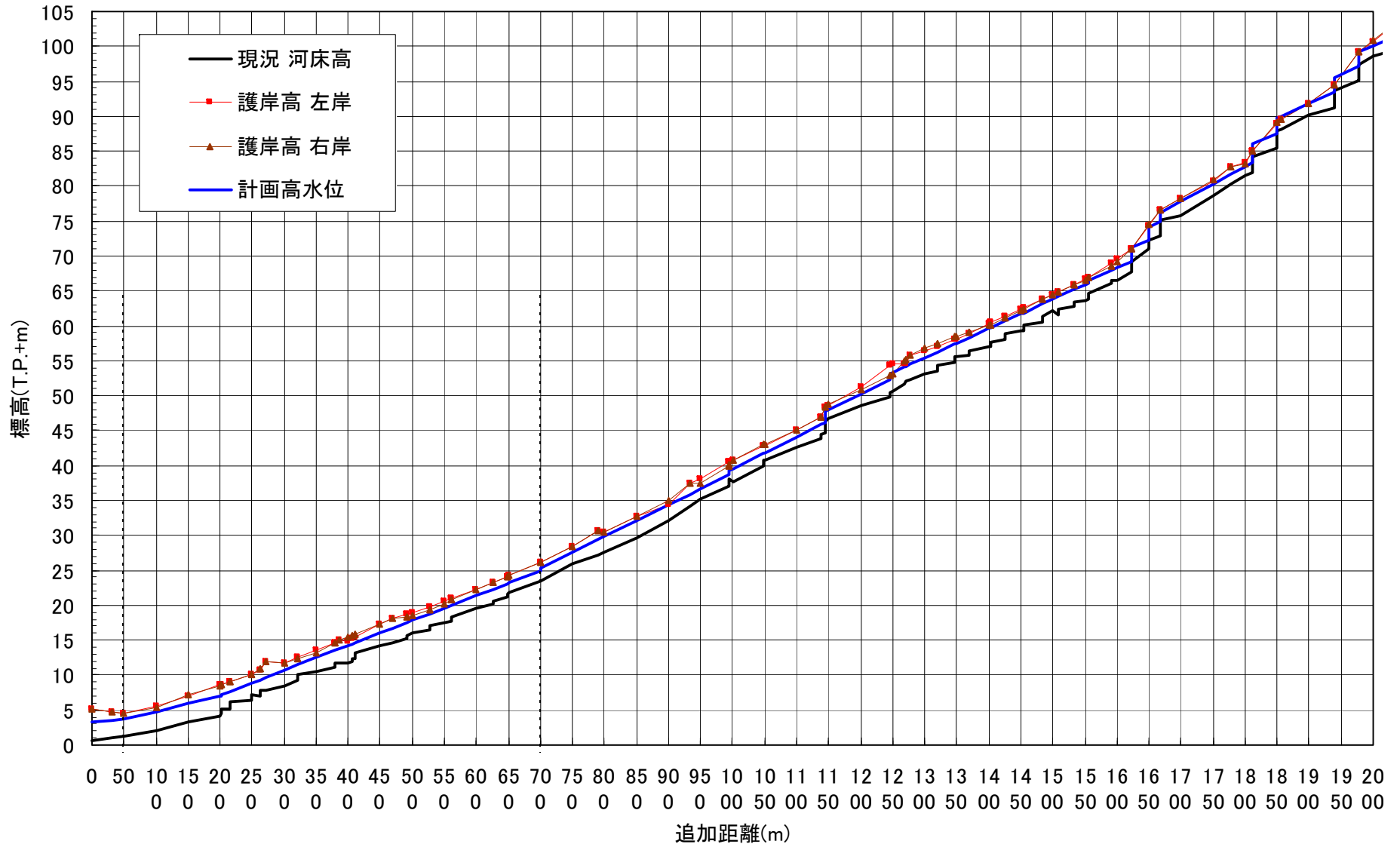
伊東宮川計画縦断面図
