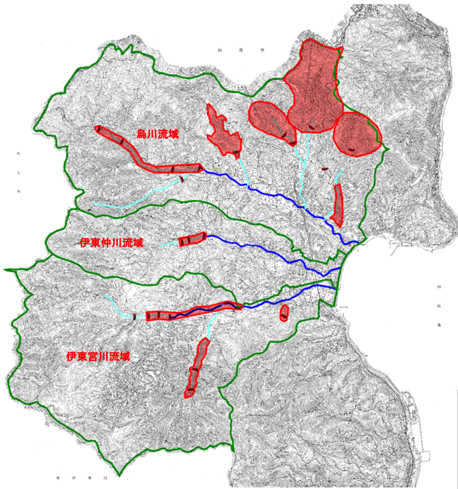
図-2.5 砂防施設位置図（宇佐美地区）
