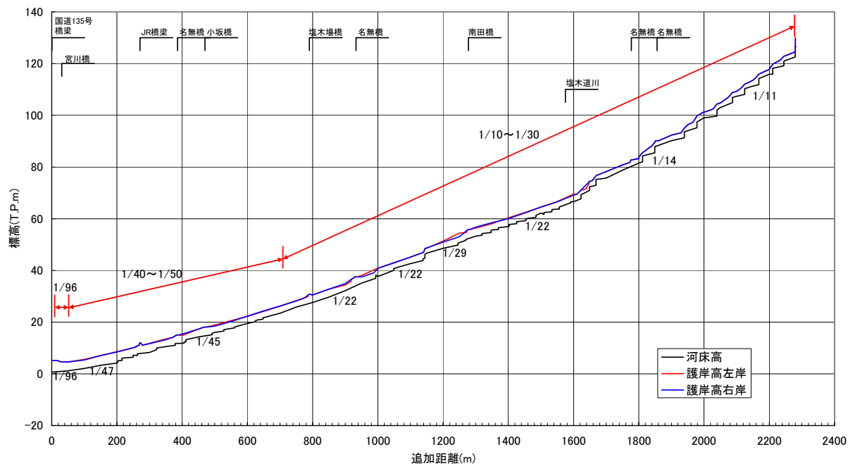
図-1.4 伊東宮川 河床高縦断図
