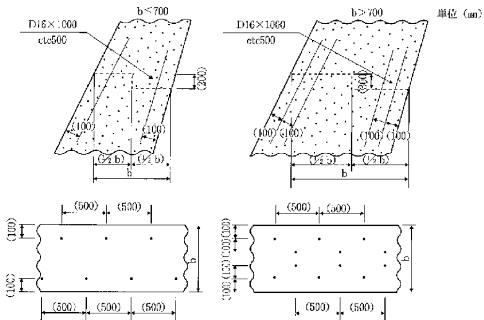
図 3-3 (水平打継目)
