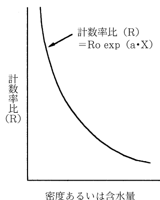
図－2 計数率比 (R) と密度および含水率の関係
