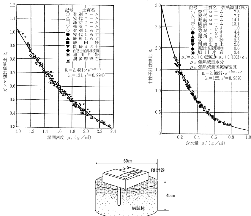
図－3 計数率比と湿潤密度および含水量の検定例
