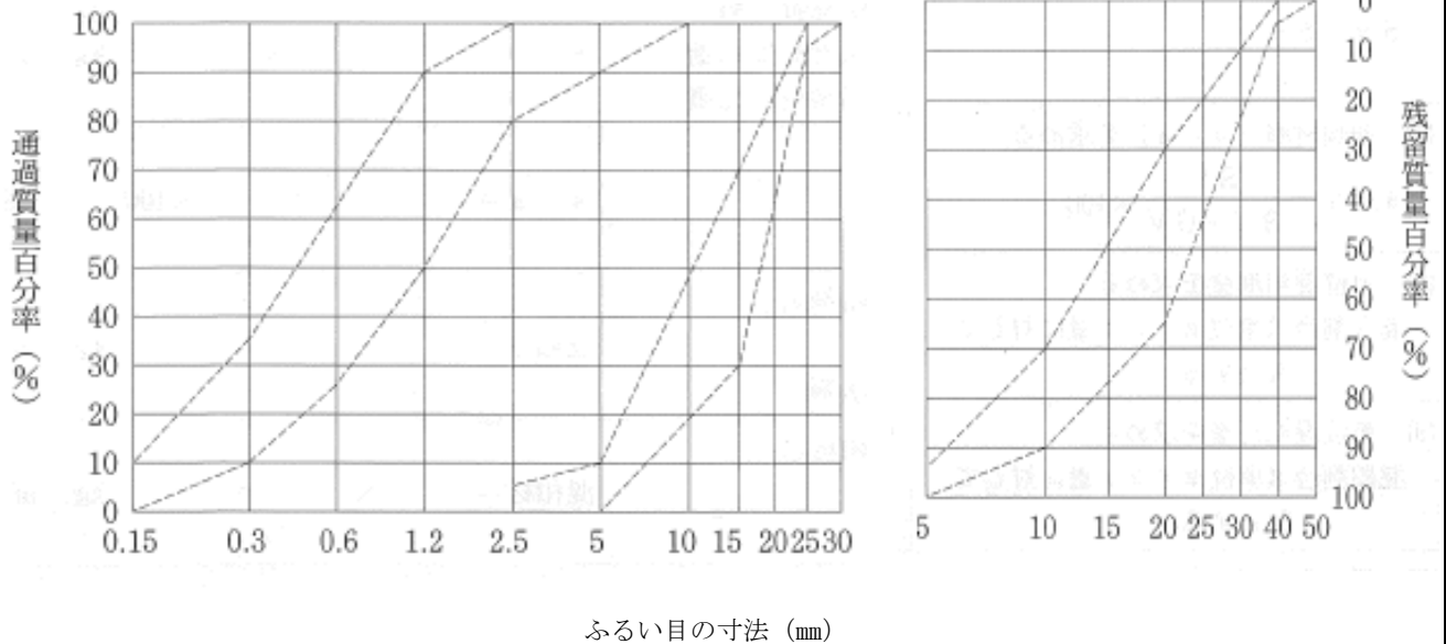
粒度曲線
