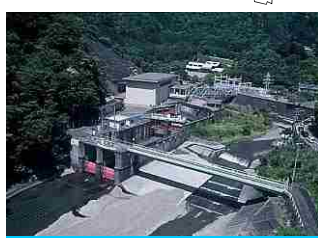
大井川用水 (川口取水工)
