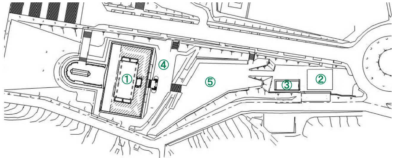
AOI-PARC配置図
