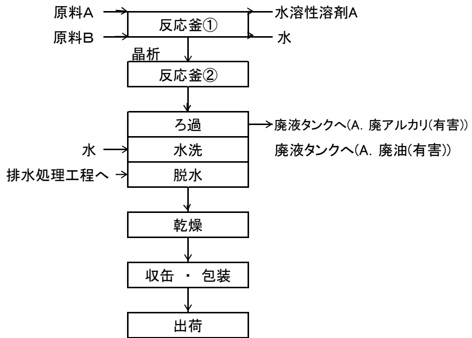
図1 半導体用感光性化学品製造フローシート
