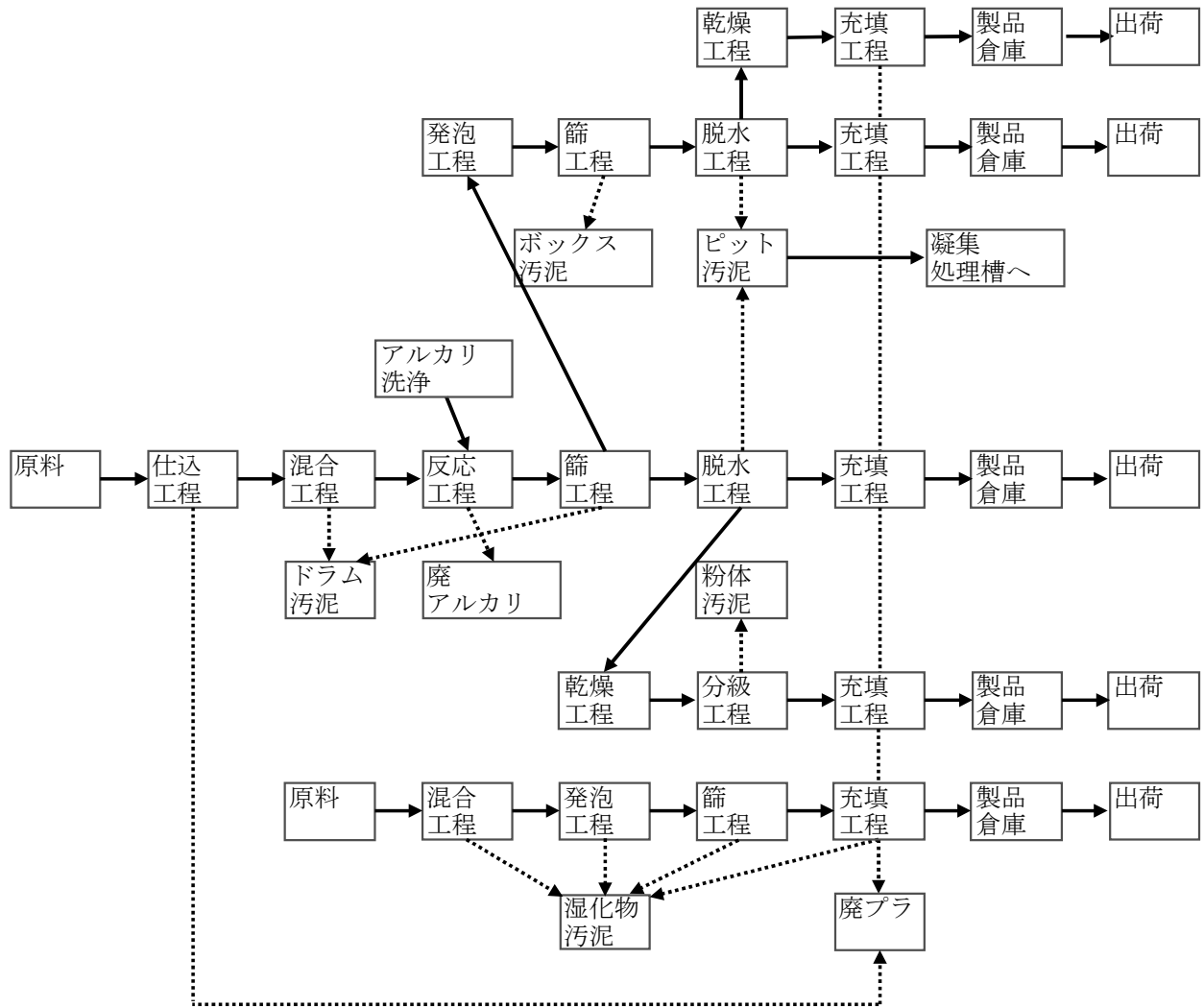
図4 マイクロカプセル製造フローシート [No.4]
