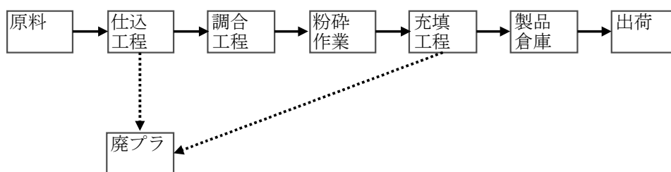
図2 生ゴム離型剤製造フローシート [No.2]
