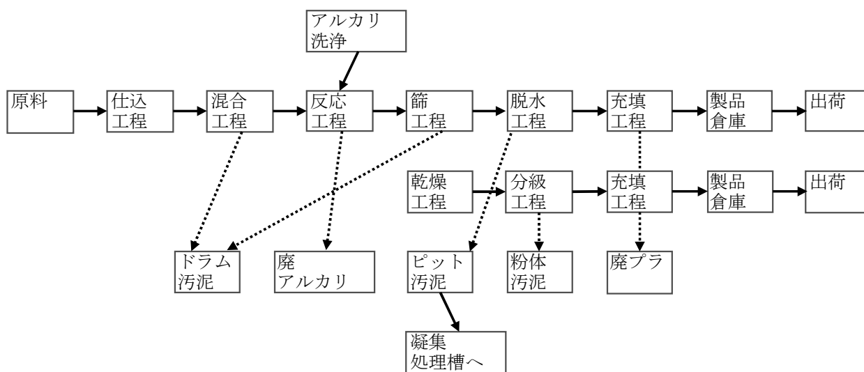
図3 プラスチック粉体製造フローシート [No.3]
