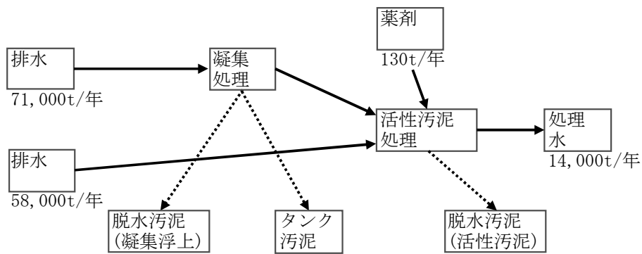
図5 排水浄化処理フローシート [No.5]
