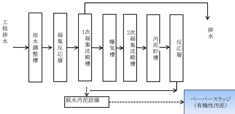
【図2】排水処理フローシート
