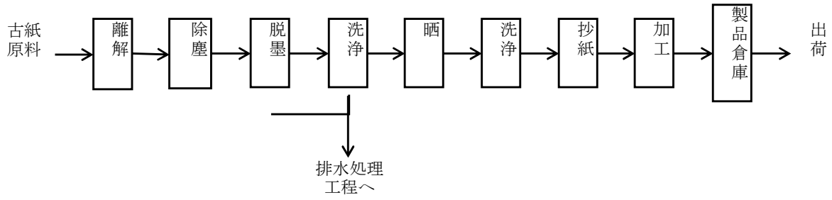
【図1】紙製造フローシート
