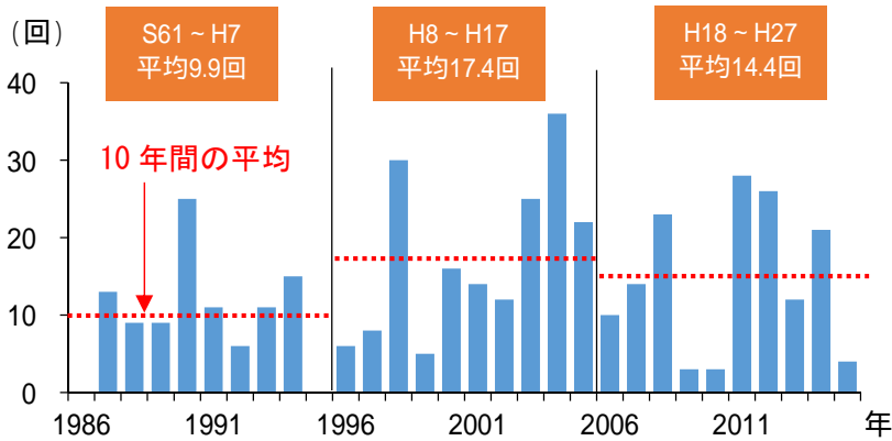
静岡県における時間雨量 50mm 以上の降雨発生回数
