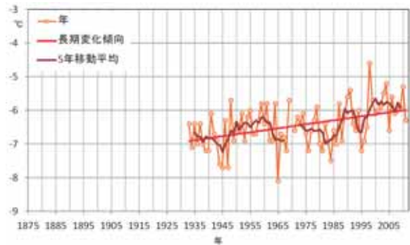
年平均気温（富士山特別地域気象観測所）
