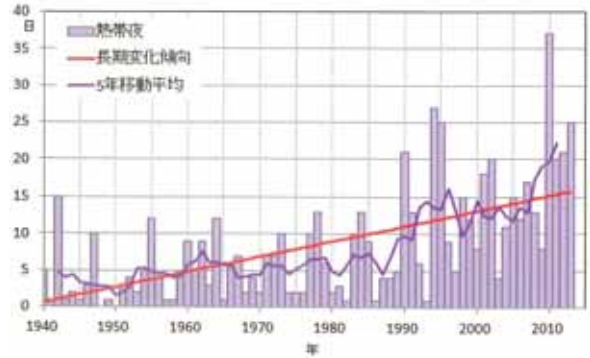
熱帯夜（日最低気温 25℃以上の日）の日
