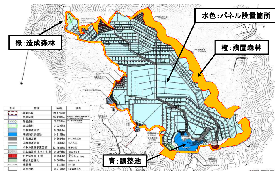
2 南伊豆町 森林地域の縮小 (太陽光発電施設) 計画平面図
