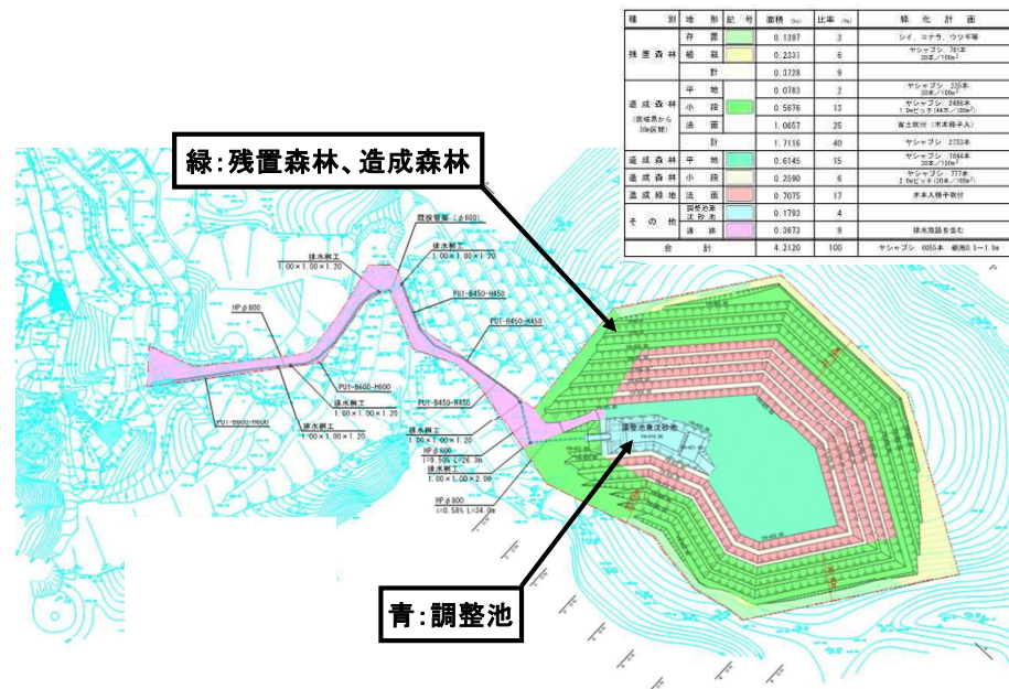
1 伊東市 森林地域の縮小（土石の採掘） 計画平面図
