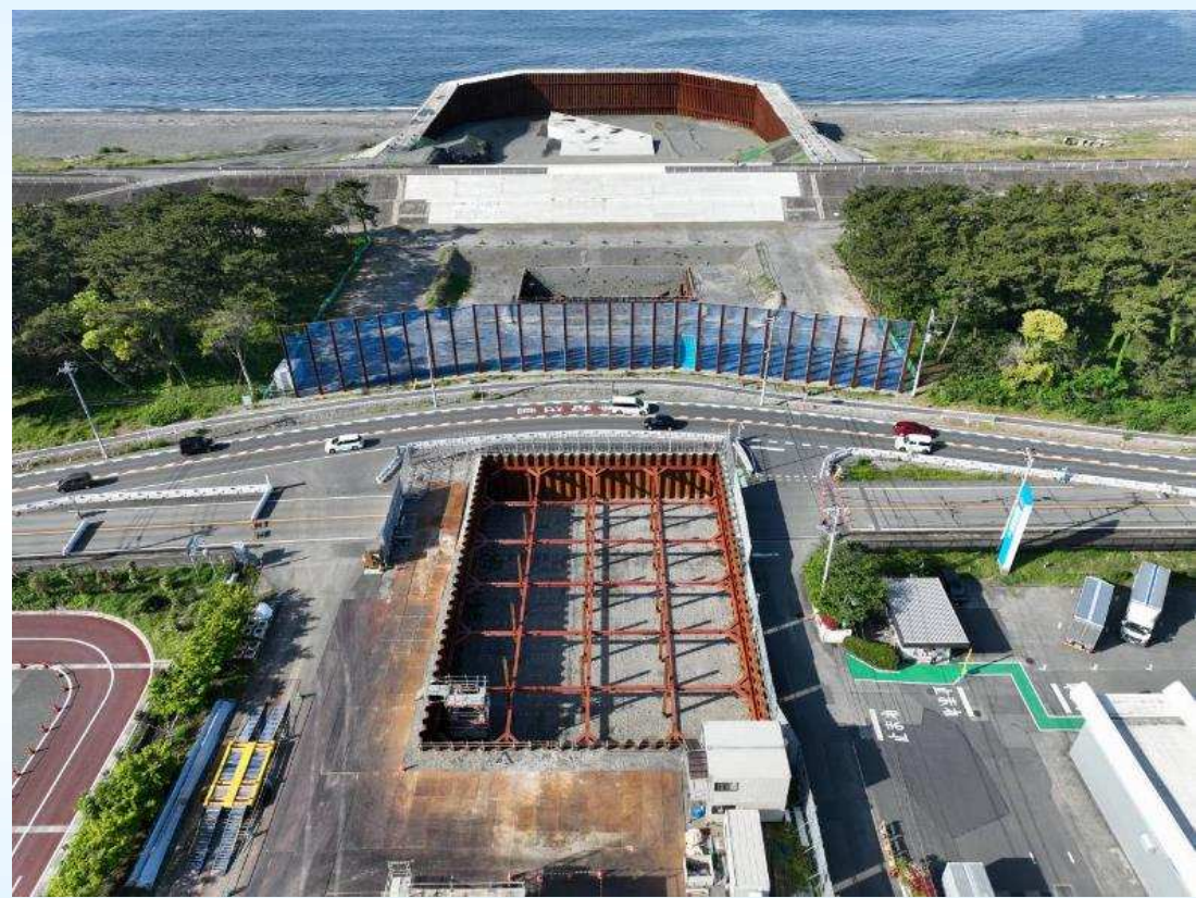
函体工(県道交差部)
