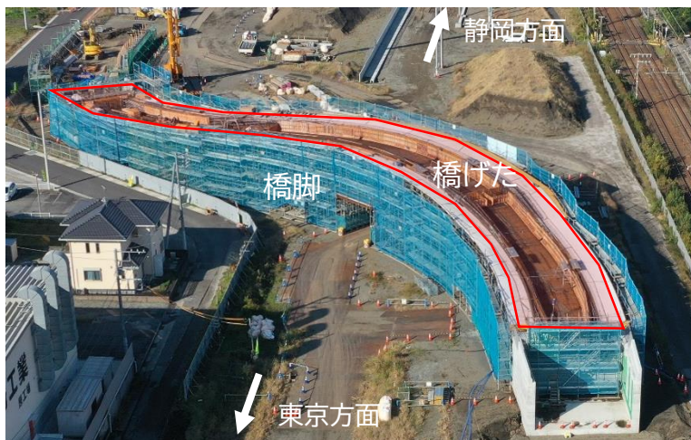
②構内跨線橋橋げたコンクリート流し込みの様子(R6.12月撮影)
